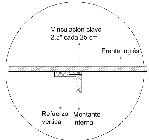
DETALLE B en planta
