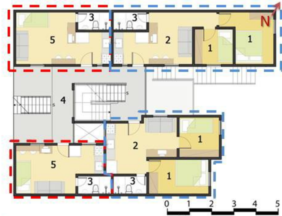
● PLANTA BAIXA – PRÉDIO DOS FUNDOS (A)
